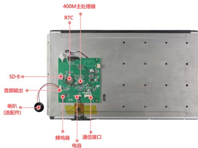
图 1-2 硬件配置图
